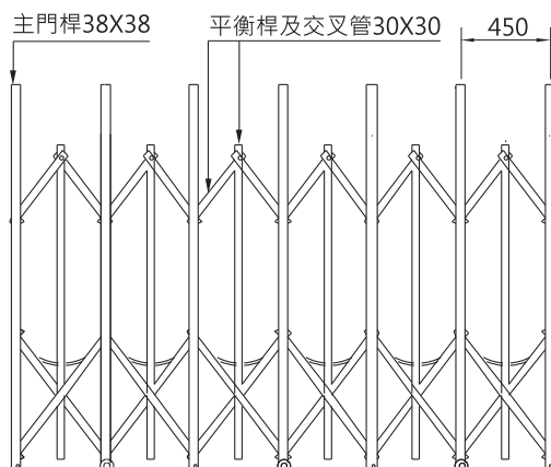
材料規格
