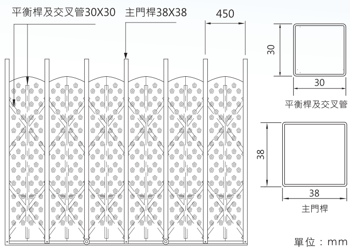
材 料 規 格
