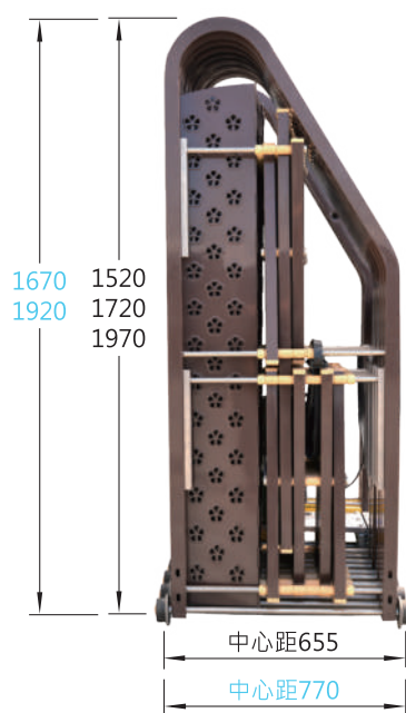
側 面 圖
