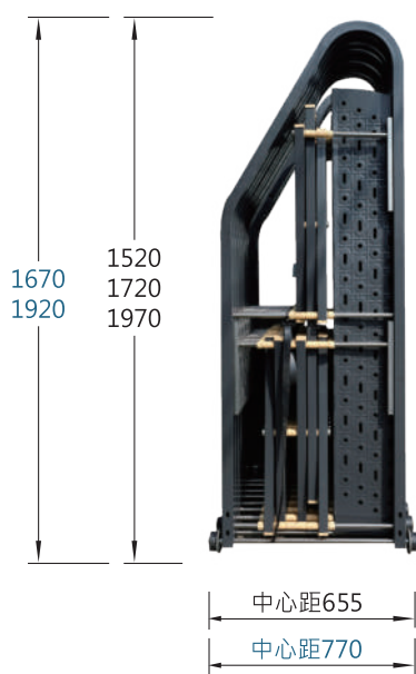
側面圖
