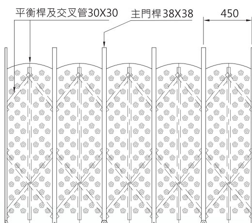
材料規格
