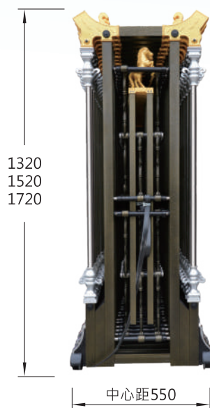
側面圖
