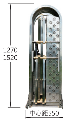
側面圖
