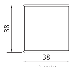
主門桿
