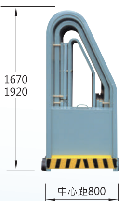
側面圖
