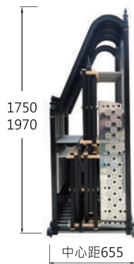
側面圖
