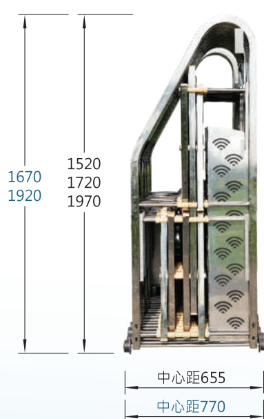
側面圖
