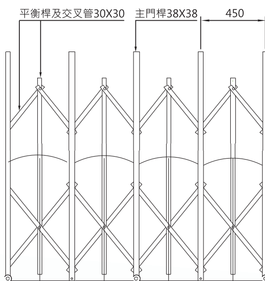
材料規格
