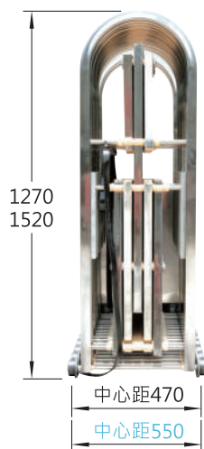
側面圖
