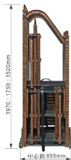
側視圖
