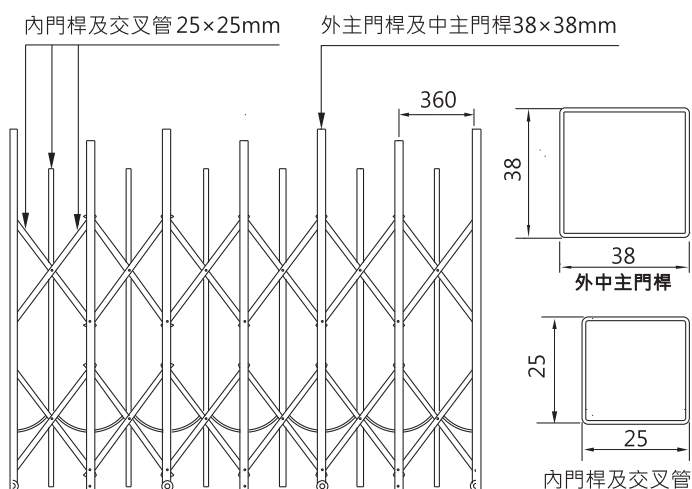
材料規格
