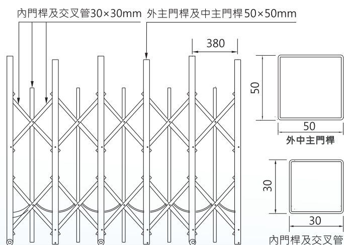
材料規格
