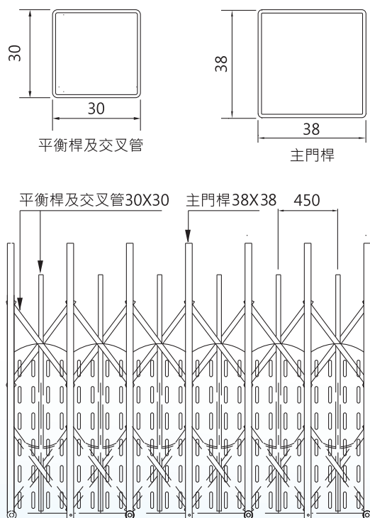
材料規格
