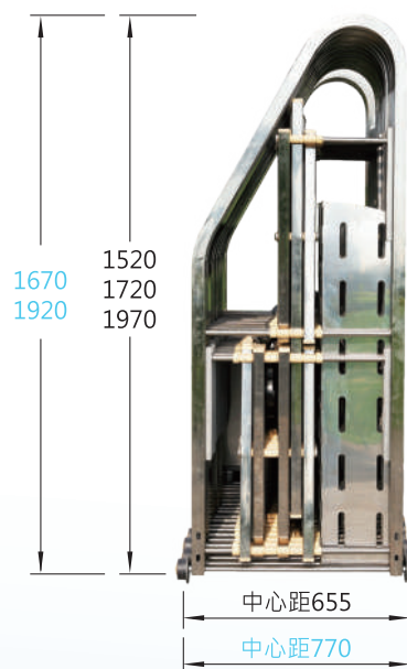
側面圖
