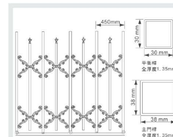
材料規格玫瑰管
