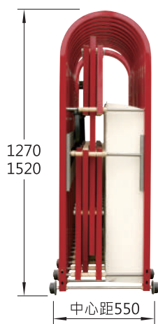
側面圖
