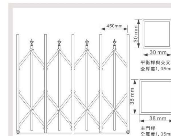
材料規格
