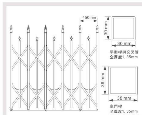
材料規格
