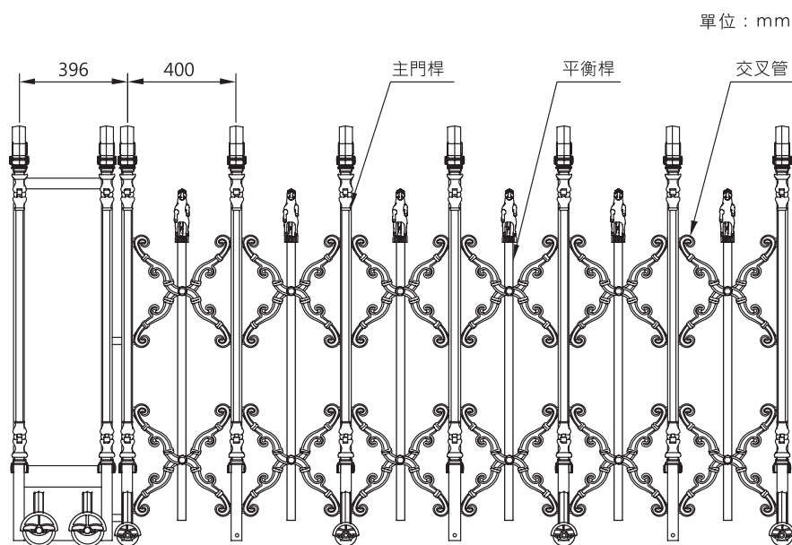
材料規格
