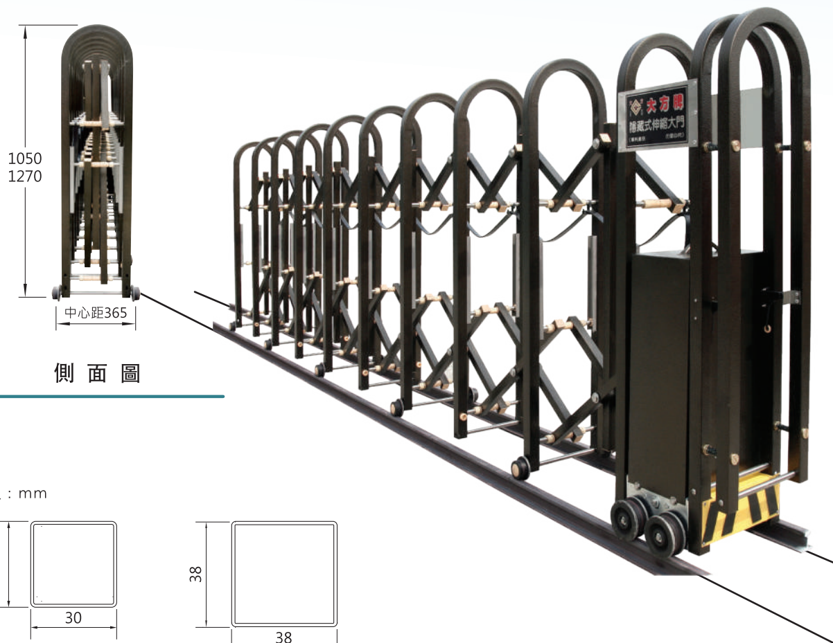
平衡桿及交叉管
