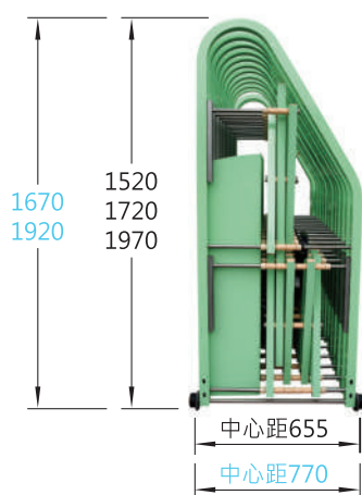
側面圖
