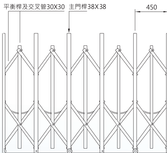
材料規格
