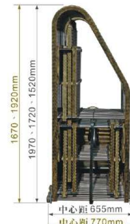
側視圖
