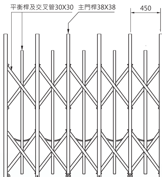
材料規格
