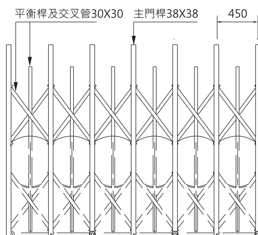
材料規格
