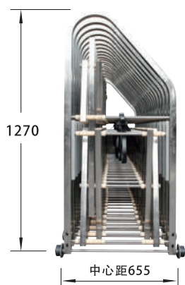
側面圖
