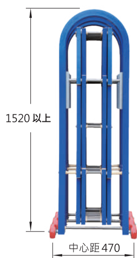
側面圖
