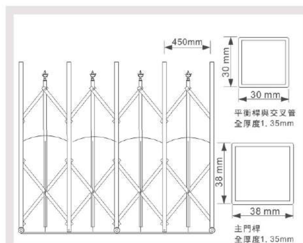
材料規格
