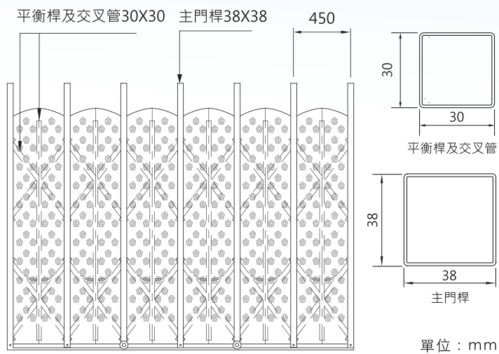
材料規格
