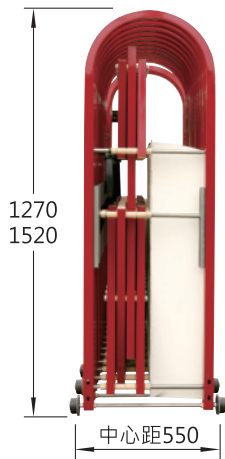
側面圖
