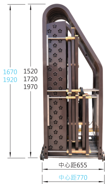
側面圖
