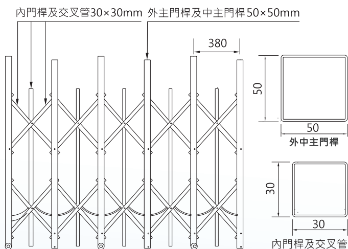
材料規格
