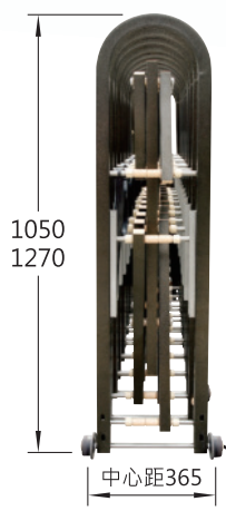
側面圖
