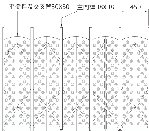
材料規格
