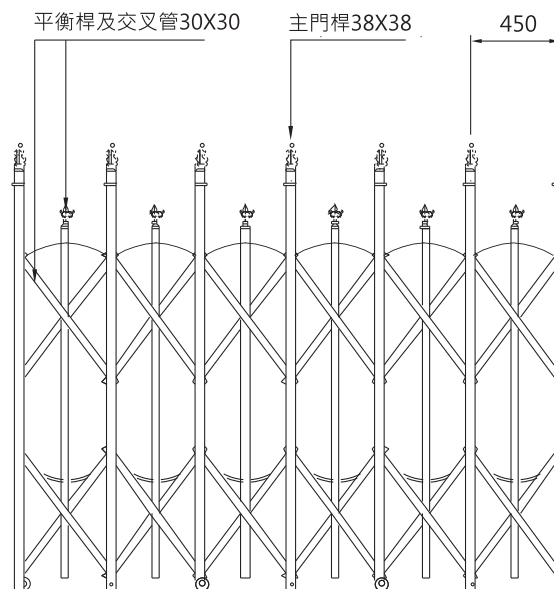
細部圖
