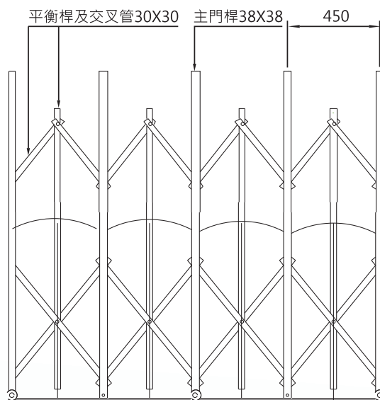
材料規格
