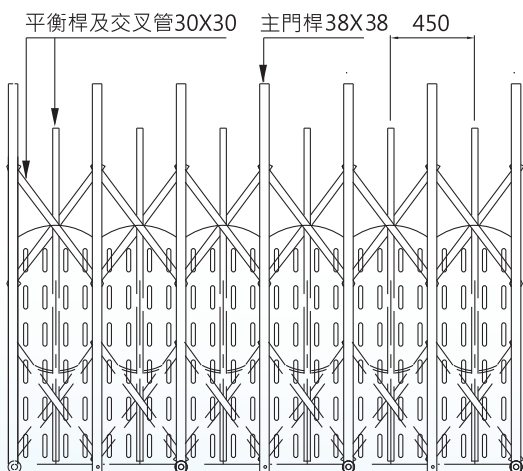
材料規格
