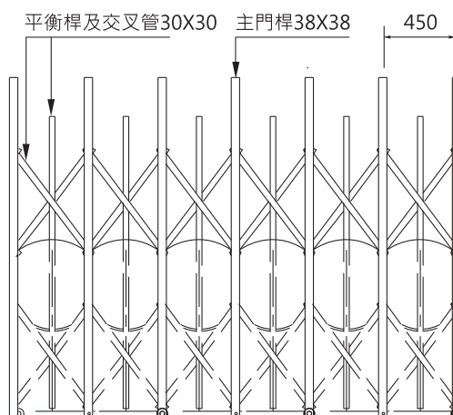
材料規格
