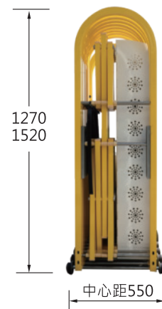
側面圖
