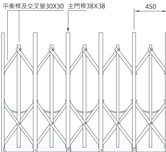
材料規格
