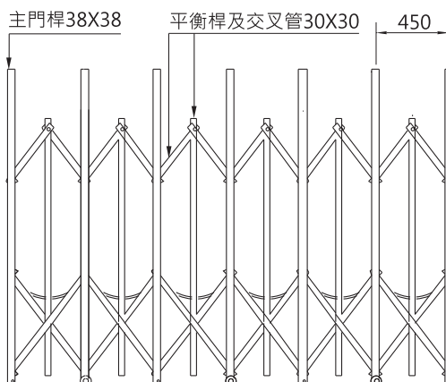
材料規格
