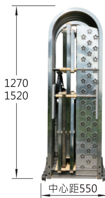
側面圖
