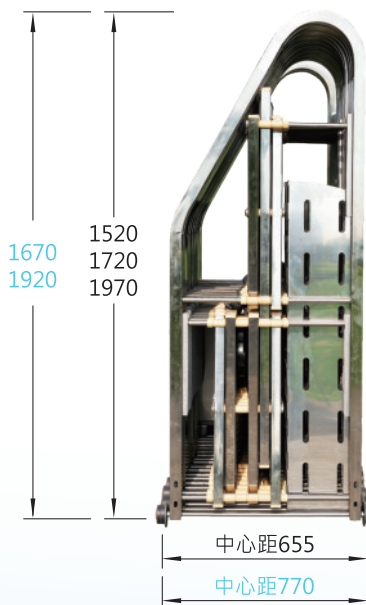
側面圖
