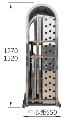
側面圖
