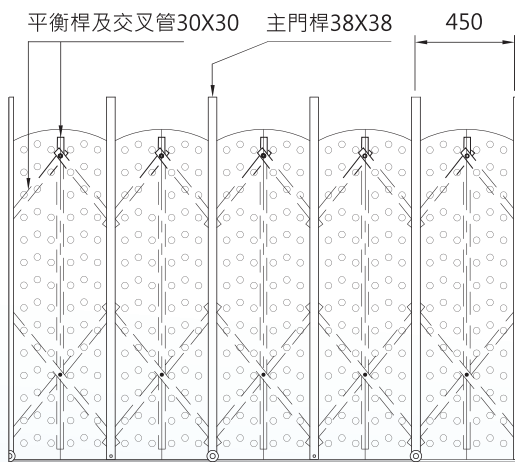
材料規格
