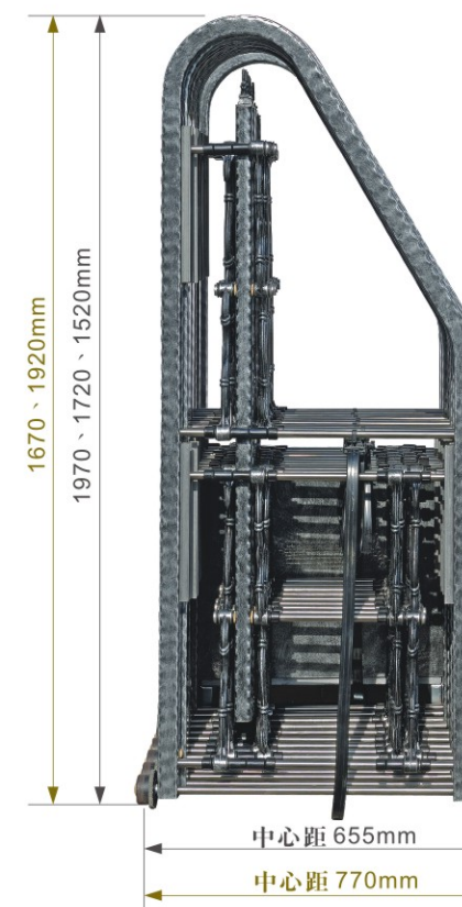
側視圖
