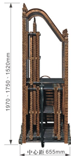
側視圖
