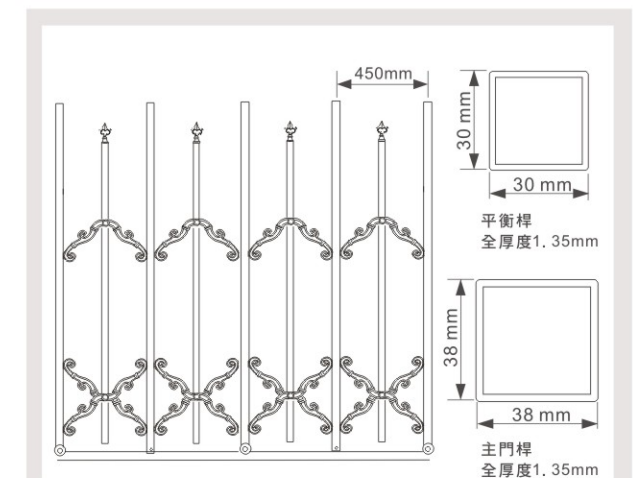
材料規格 - 玫瑰管
